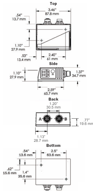
QX-830 Dimensions
